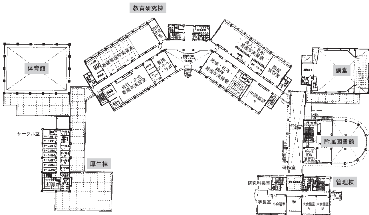
4) 校舎2階平面図
